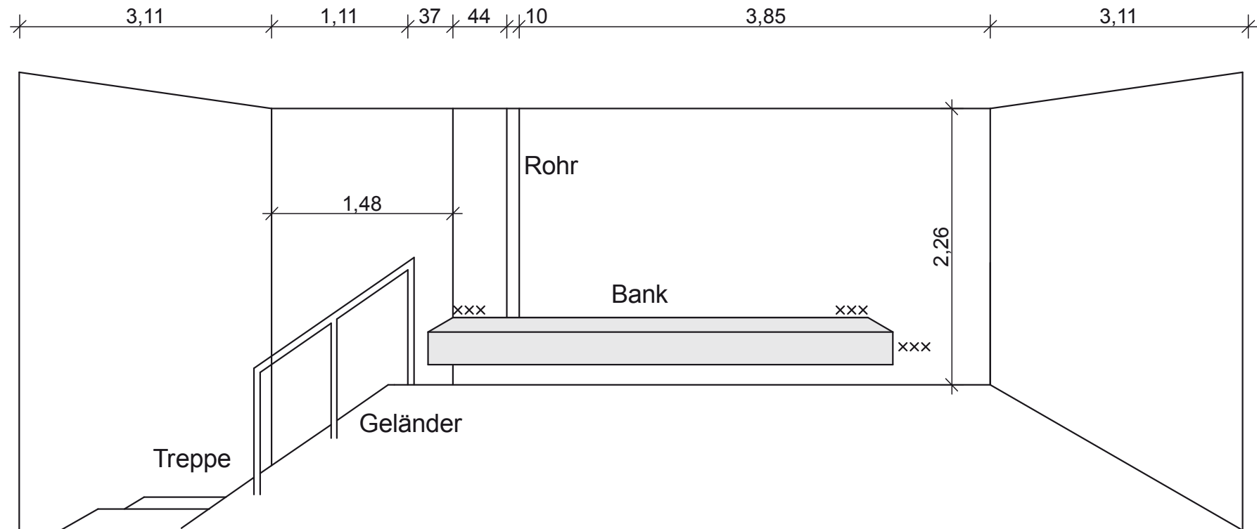
Wandabwicklung (nicht maßstabgerecht)
